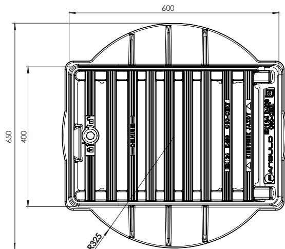
RYSUNEK POGLĄDOWY
