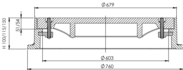
RYSUNEK POGŁĄDOWY
