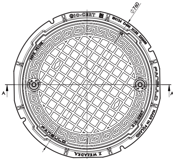
RYSUNEK POGŁĄDOWY
