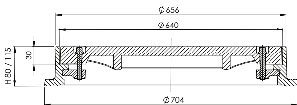
RYSUNEK POGLĄDOWY
